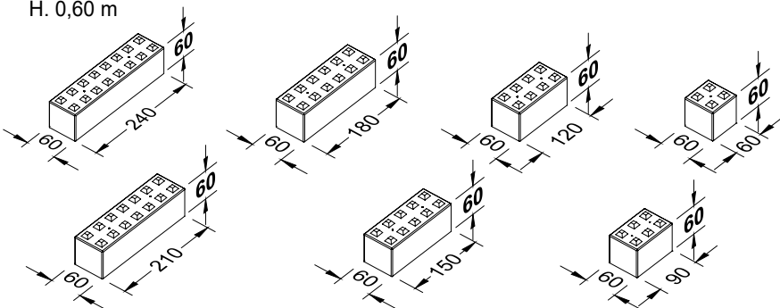
NUT-UND FEDER STEIN H. 0,60 m
