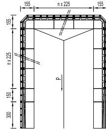
EINFACHER SILO
