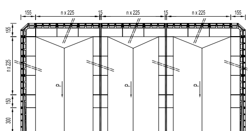
SILOSI POSTAVLJENI DRUG OB DRUGEM
