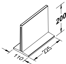
PREGRADEN SUPER H. 2,00 m
