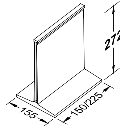
PREGRADEN H. 7,00 m H. 8,00 m H. 9,00 m
