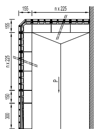
SILO POVEZAN Z ŽE OBSTOJEČO STENO
