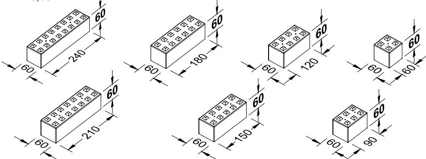
BLOKIRNA OPEKA H. 0,60 m
