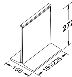
DIVISORIO H. 7,00 m H. 8,00 m H. 9,00 m
