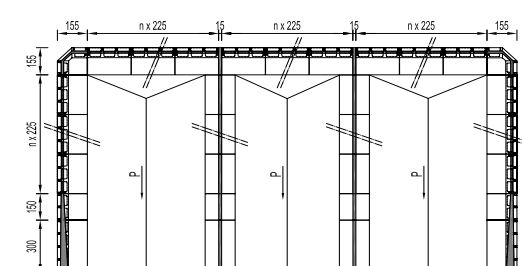
SILOS AFFIANCATI
