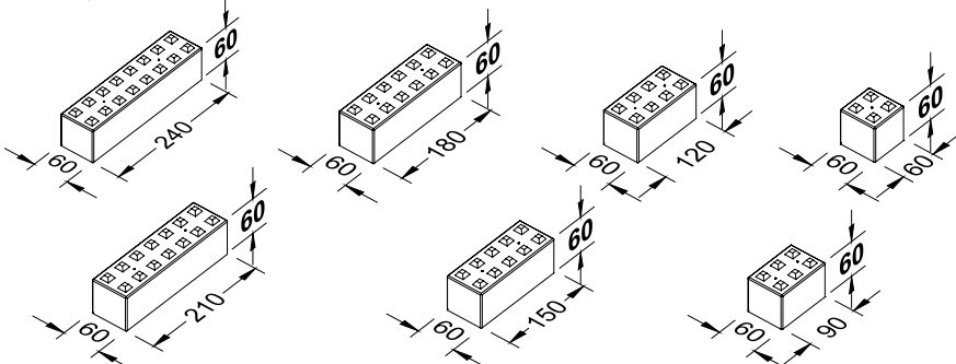
BLOCCO INCASTRO H. 0,60 m
