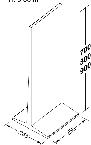
DIVISORIO H. 7,00 m H. 8,00 m H. 9,00 m
