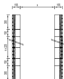
SILO SEMPLICE APERTO
