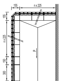
SILO IN ADERENZA A MURO ESISTENTE
