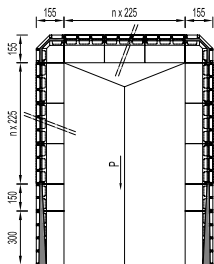
SILO SEMPLICE
