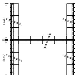
SILOS CONTRAPPOSTI
