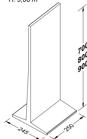
PARTITION WALL H. 7,00 m H. 8,00 m H. 9,00 m
