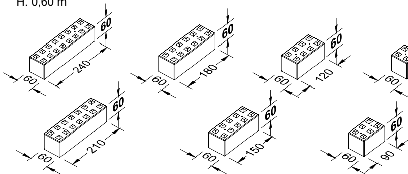
INTERLOCKING BLOCK H. 0,60 m
