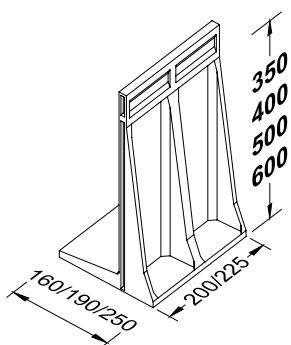
PERIMETER WALL H. 3,50 m H. 4,00 m H. 5,00 m H. 6,00 m
