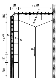
SILOS POVEZAN Z ŽE OBSTOJEČO STENO
