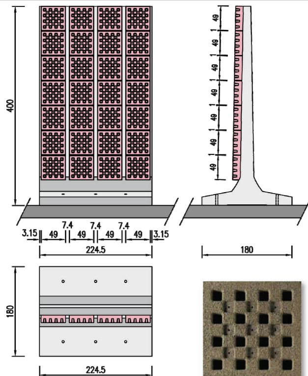
FONOLECA QUADRO DIMENSIONE MODULO 50X50 cm
