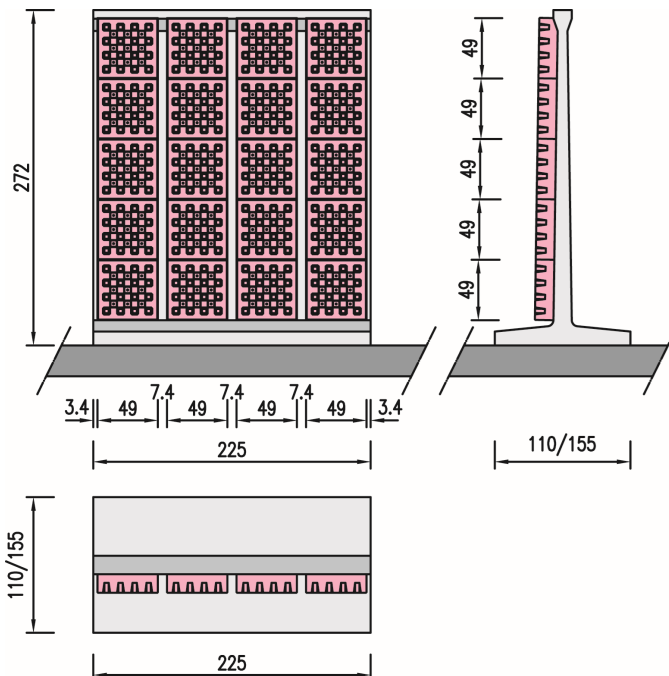
FONOLECA QUADRO DIMENSIONE MODULO 50x50 cm
