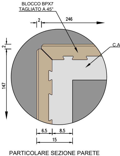
PARTICOLARE SEZIONE PARETE
