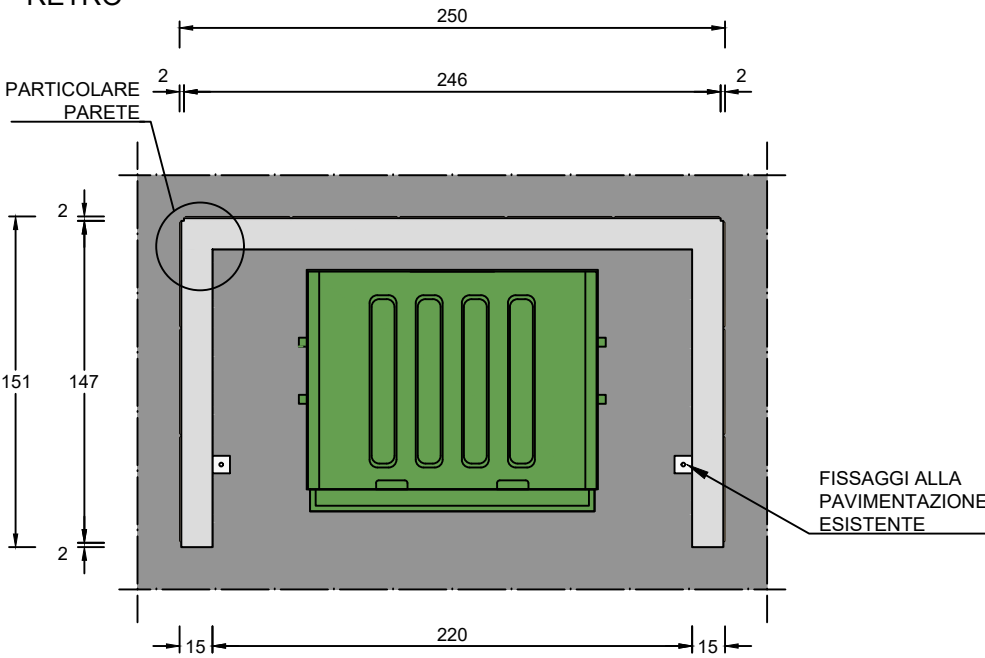
PIANTA
