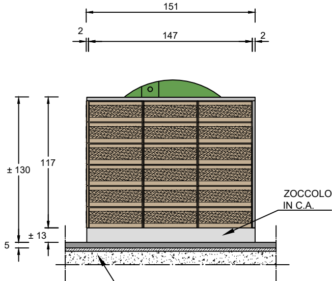
PROSPETTO LATERALE
