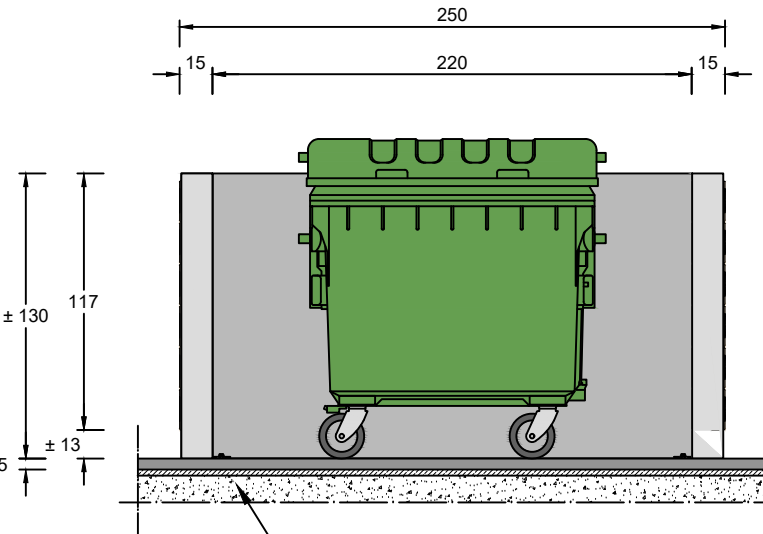
PROSPETTO FRONTALE
