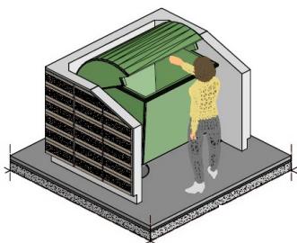
Box "A" / "B" dim. 200/250 x 150 (1 pannello)
