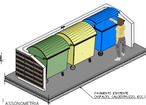
Box "D" dim. 495 x 150 (2 pannelli)
