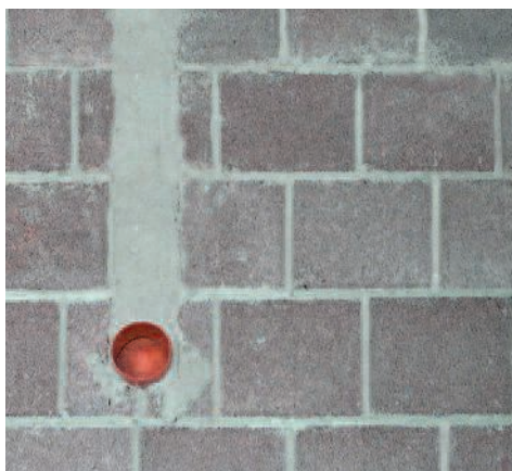
Parete divisoria con ponte acustico dovuto alla presenza di cavedio impiantistico.
