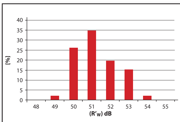
Figura 1: Distribuzione percentuale dei valori di R'_w misurati per le pareti realizzate con blocchi di 25 cm di spessore.
