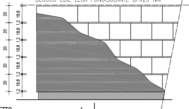
BLOCCO EDIL LECA FONOISOLANTE BFX25 NAF
