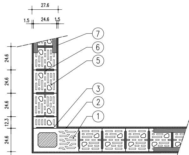
BLOCCO EDIL LECA FONOISOLANTE BFX25 NAF
