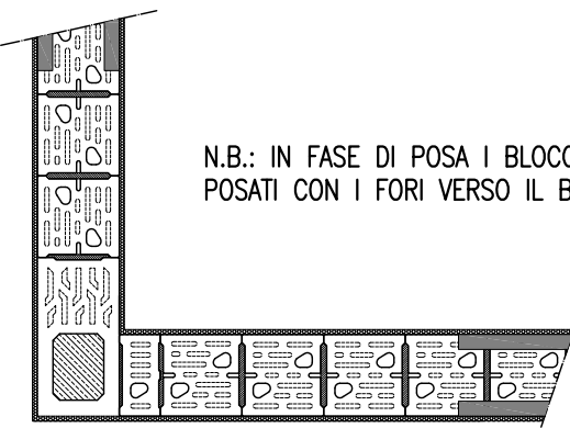
BLOCCO EDIL LECA FONOISOLANTE BFX25 NAF
