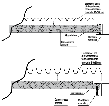
MONTANTE METALLICO A VISTA
